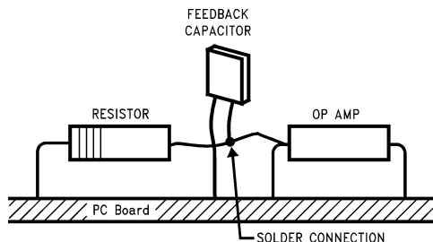
Figure 30. Air Wiring
